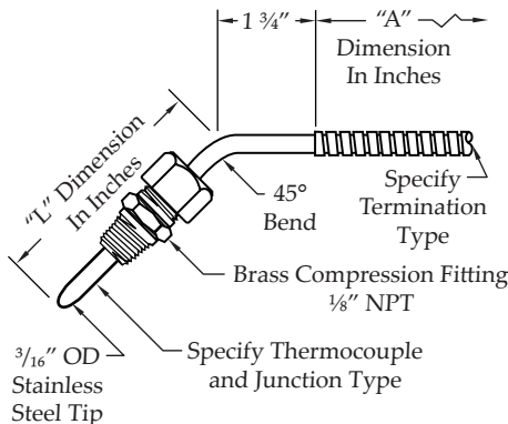
TCF45 - 45° Bend Thermocouple
